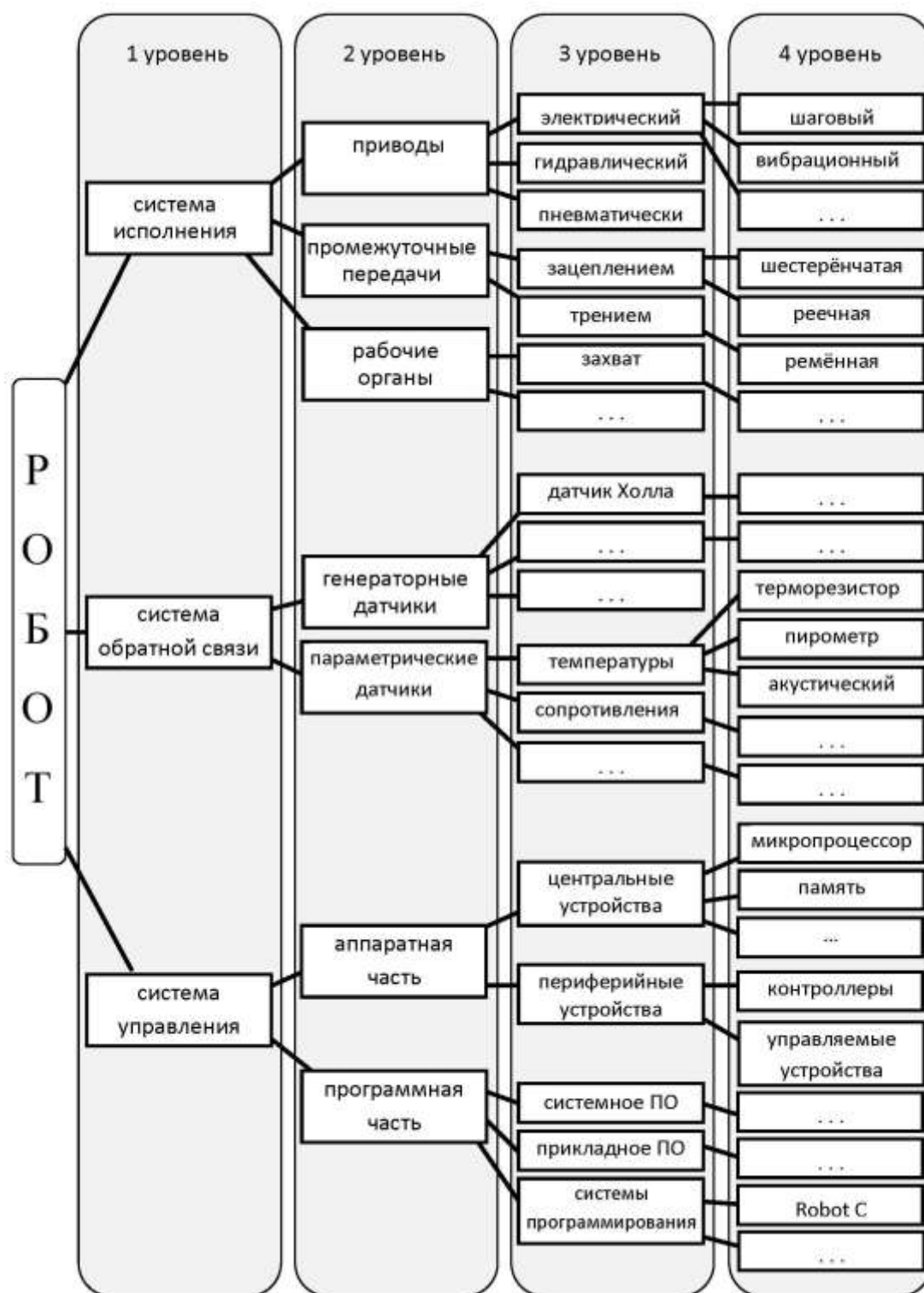
Рис. 2. Уровни рассмотрения структуры робота
