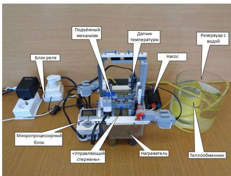
Рис. 3 Модель терморегуляции ядерного реактора и регулировки интенсивности ядерной реакции
